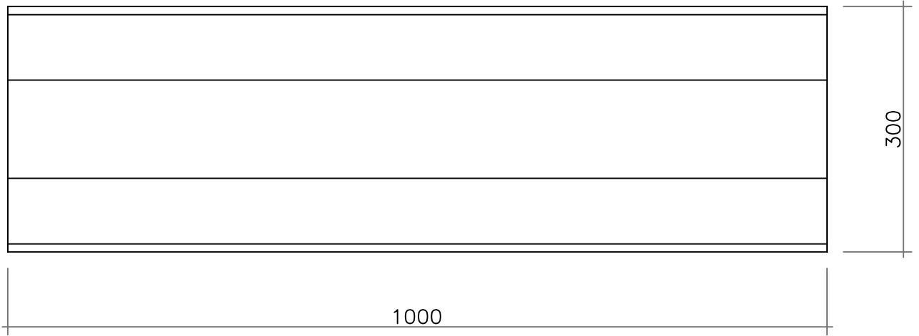
PLANTA Top View
